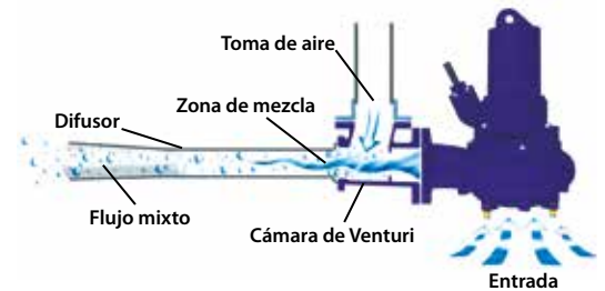
VENTURI-JET
